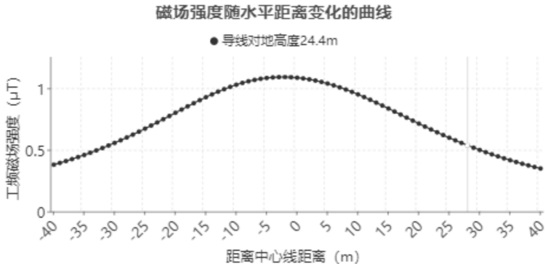
图 4-3 本项目 110kV 双回架空线路工频磁感应强度分布图
