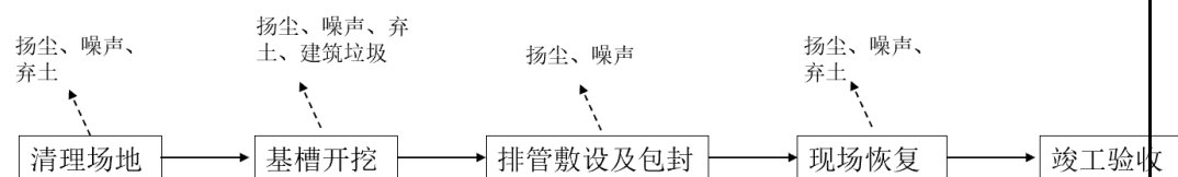
图 2-7 电缆排管施工工艺流程及产污节点图
