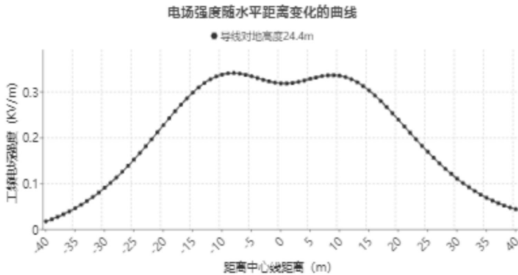
图 4-2 本项目 110kV 双回架空线路工频电场强度分布图
