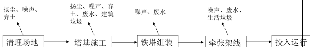
图 2-5 架空线路施工期工艺流程图
