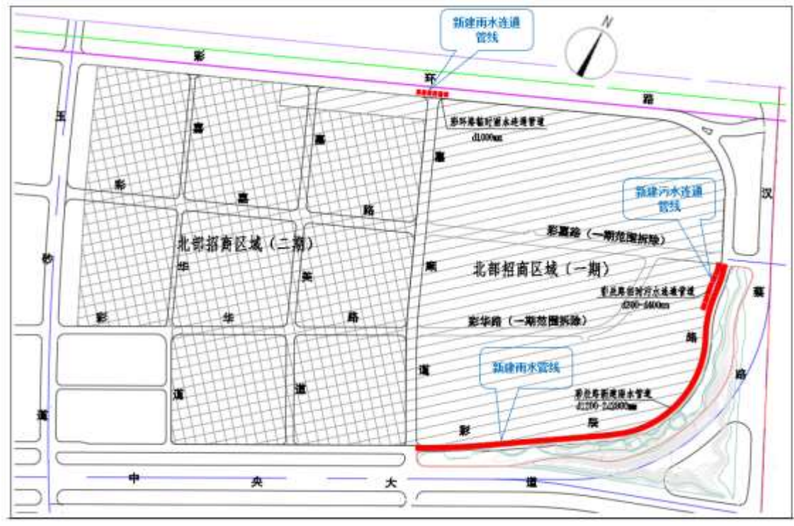
图1.1-5 本项目管线路由示意图
